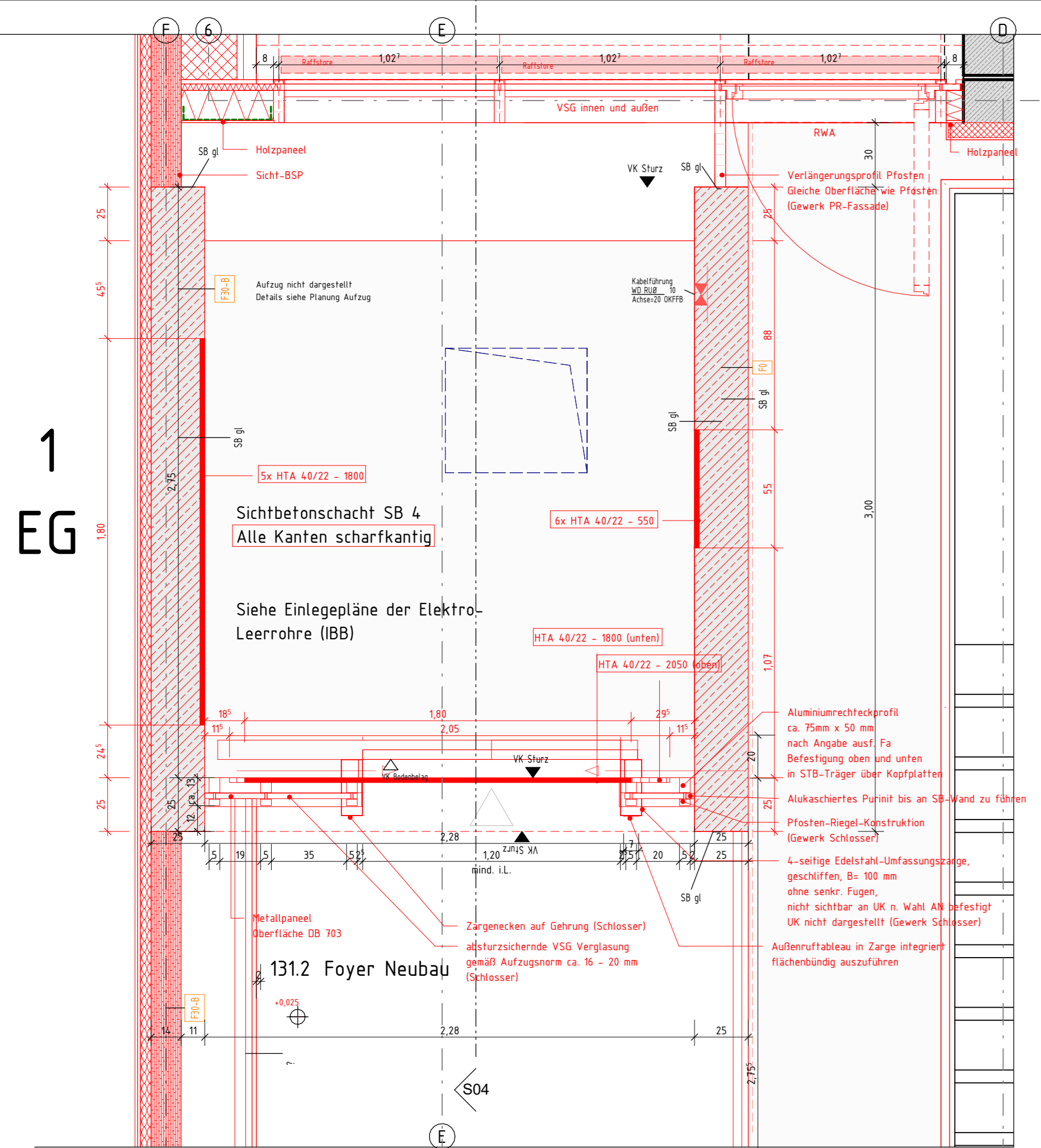
GR_Aufzug Verwaltung EG M 1 : 20
