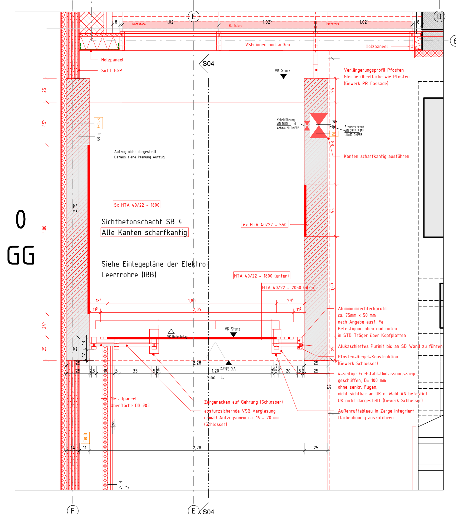
GR_Aufzug Verwaltung GG M 1 : 20
