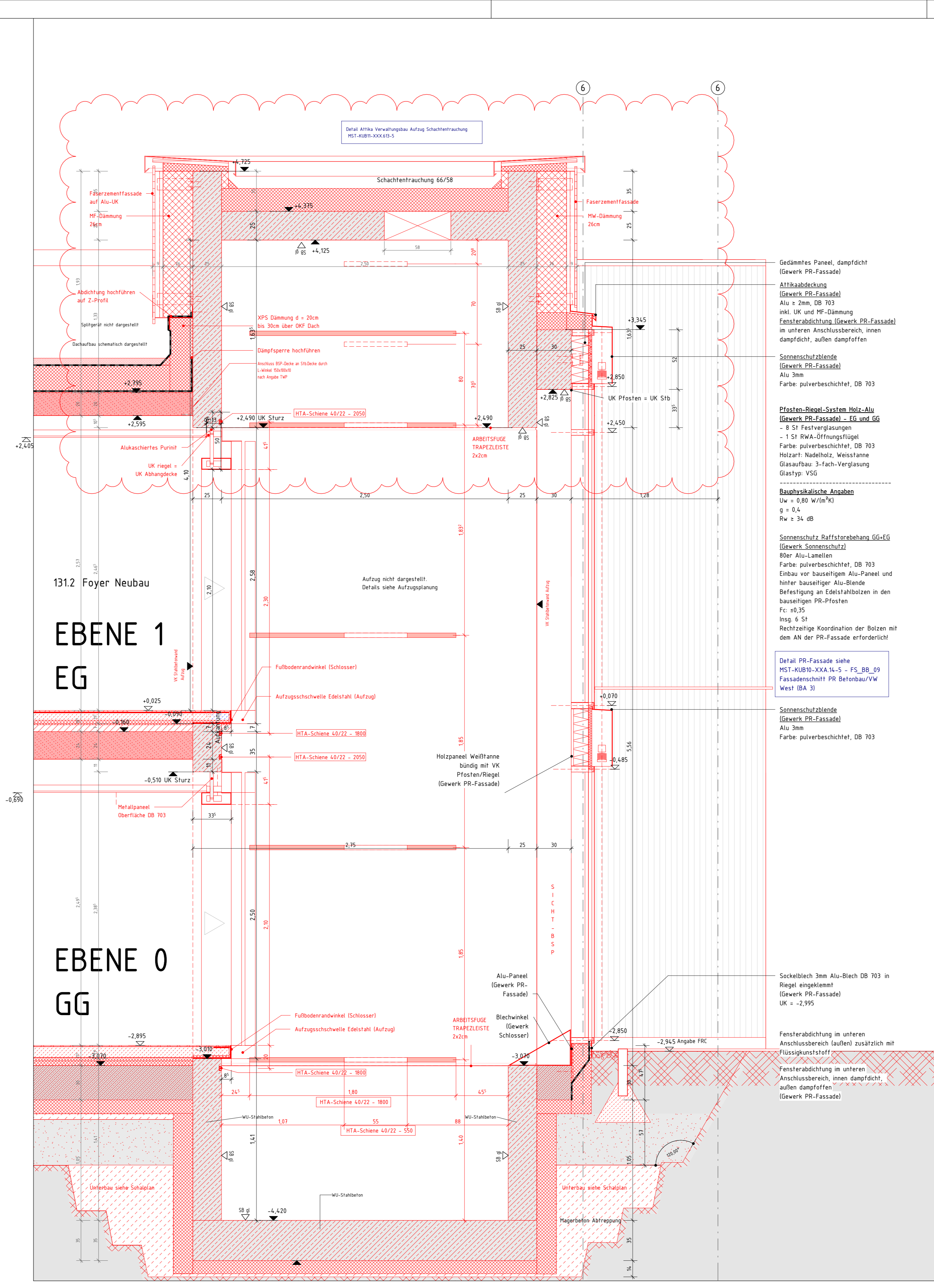
DT_SN_Aufzug Verwaltung Nord M 1 : 20
