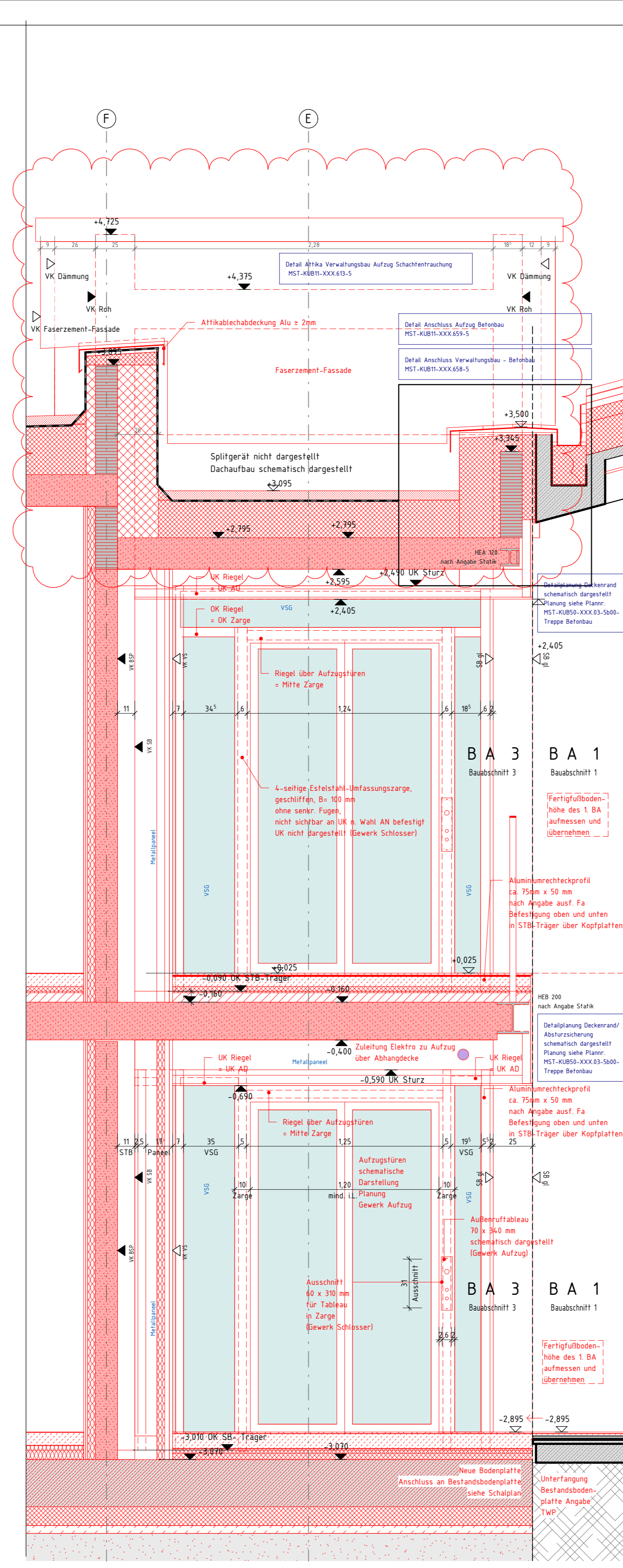
DT_AN_Aufzug Verwaltung Ost M 1 : 20
